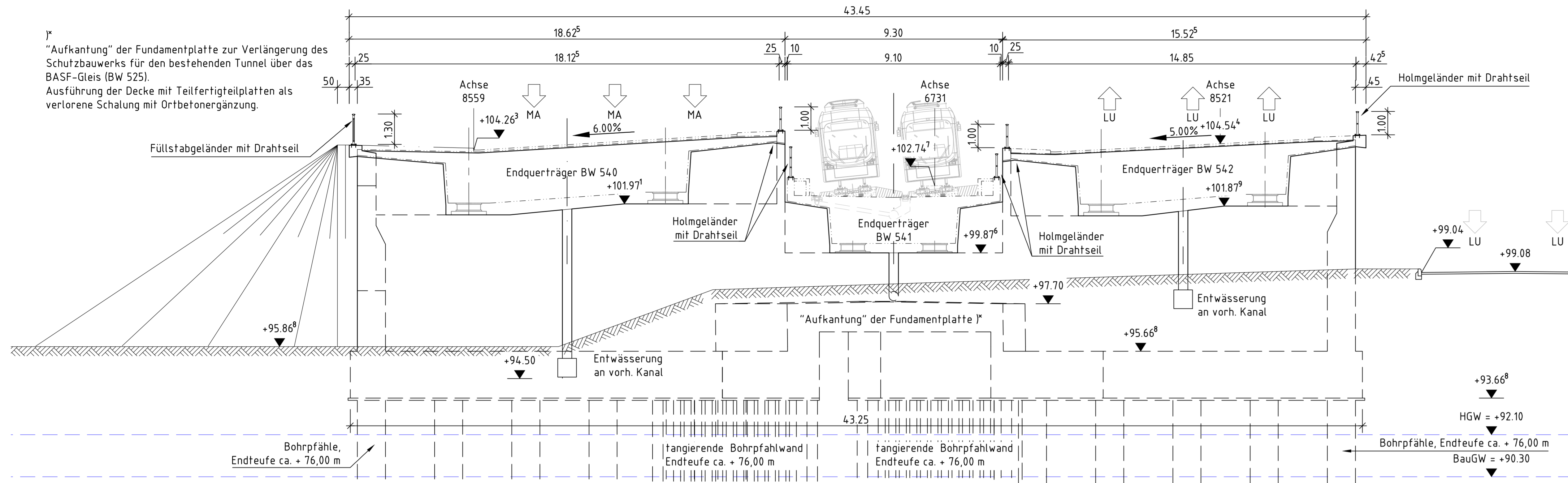
Frontansicht M 1:100
