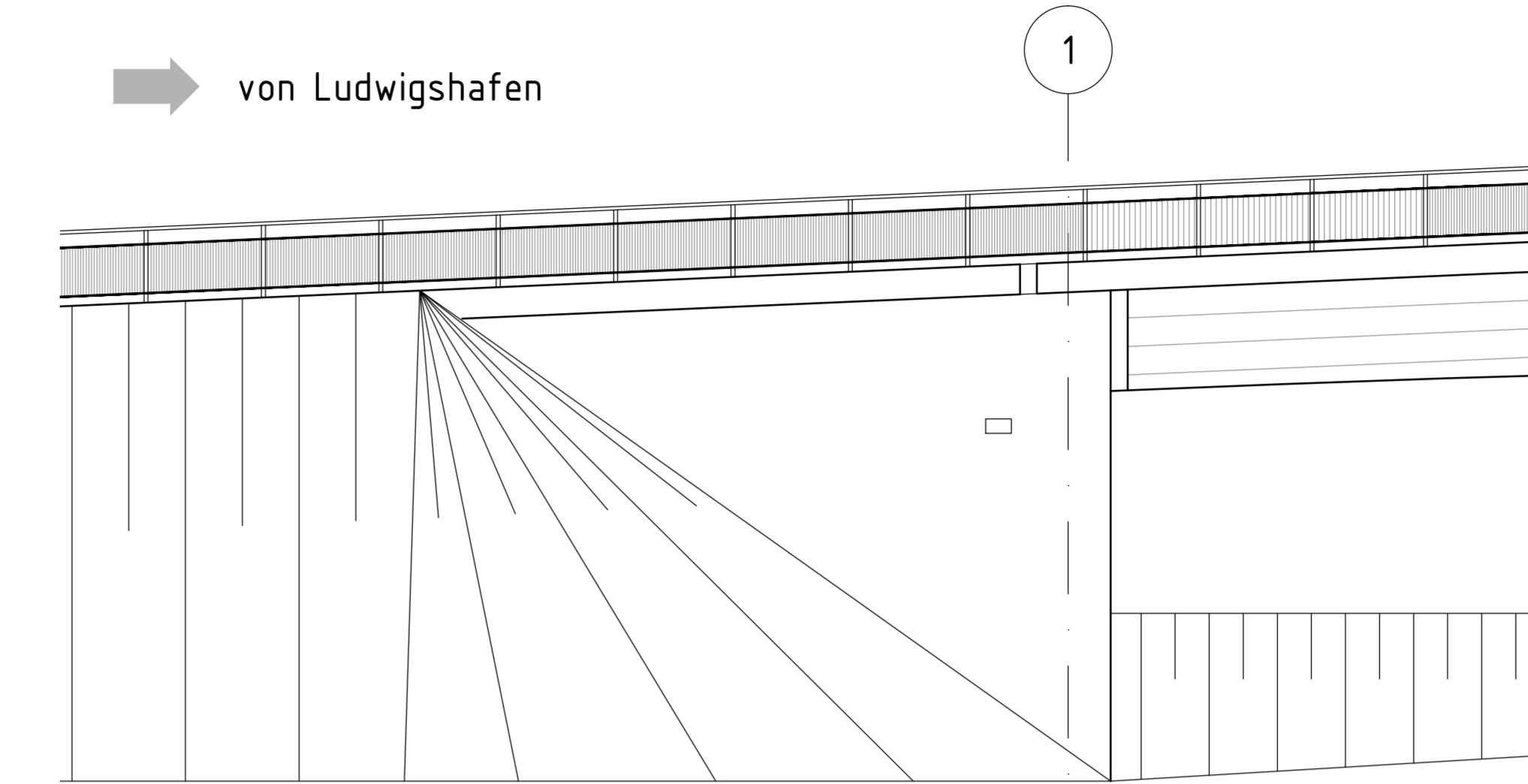
Seitenansicht Widerlager M 1:100
