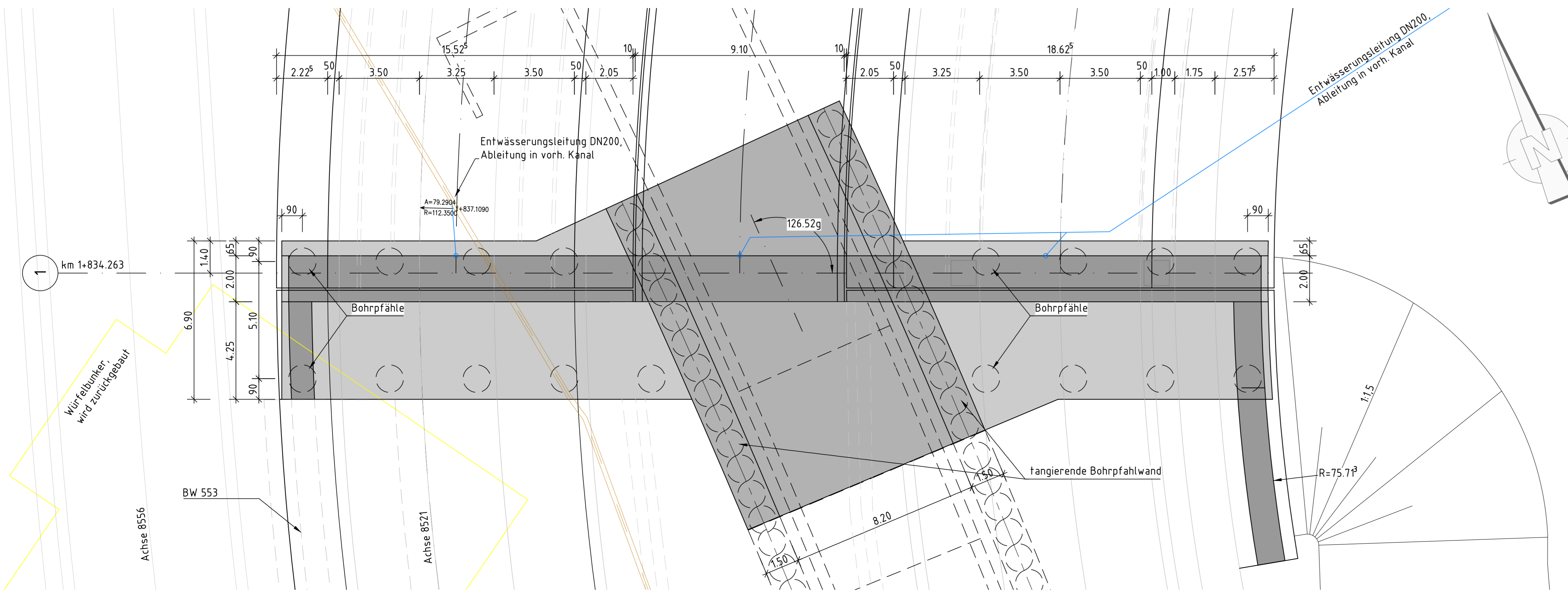
Draufsicht M 1:100
